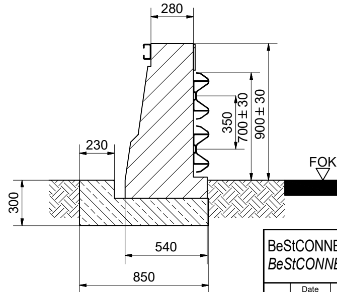
Schnitt C-C Section C-C
