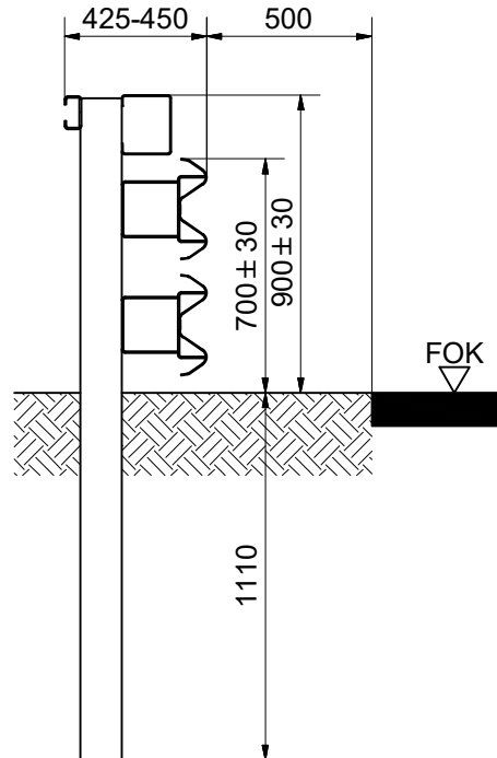
Schnitt B-B Section B-B
