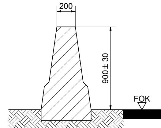
Schnitt D-D Section D-D
