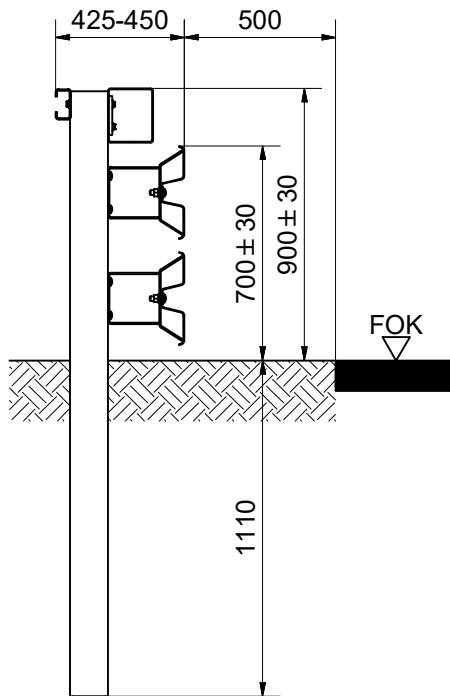
Schnitt B-B Section B-B
