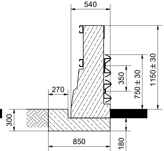
Schnitt E-E Section E-E
