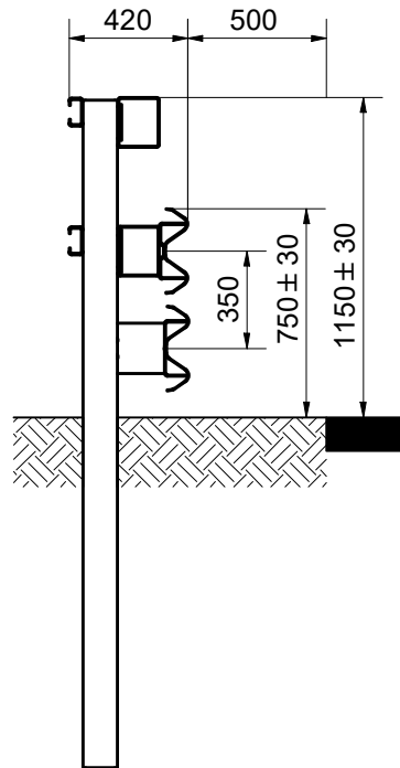
Schnitt C-C Section C-C
