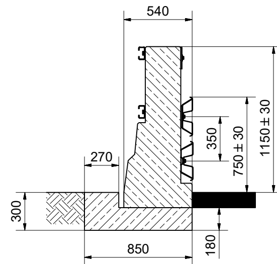
Schnitt E-E Section E-E
