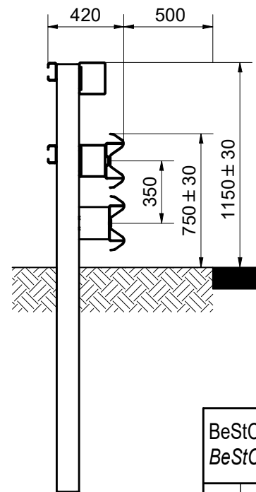
Schnitt D-D Section D-D
