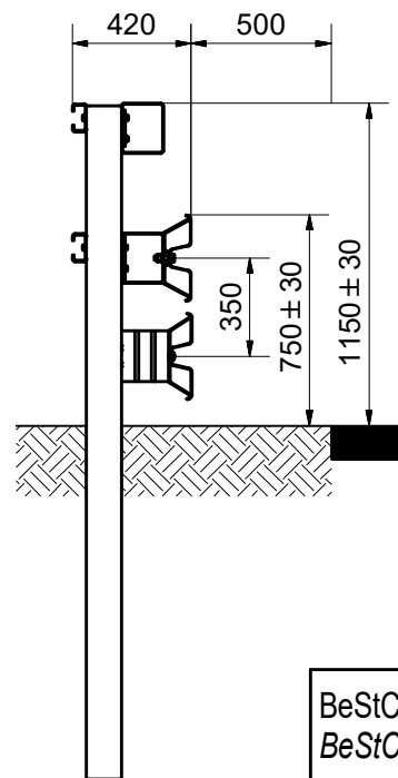
Schnitt D-D Section D-D
