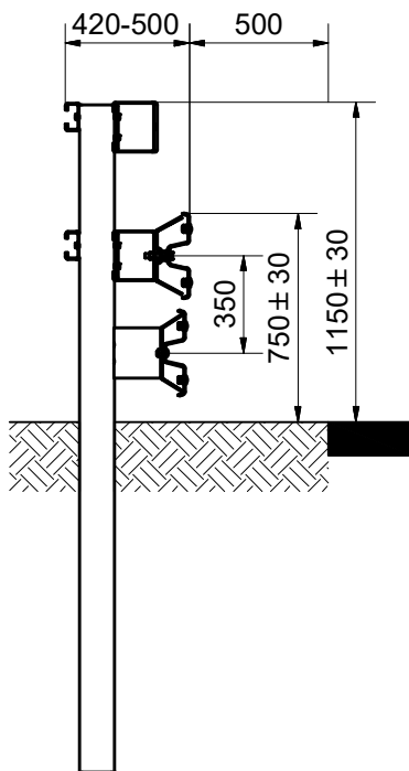
Schnitt B-B Section B-B
