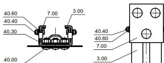
Verschraubung Abstandhalter/Pfostenklaue mit dem Pfosten
