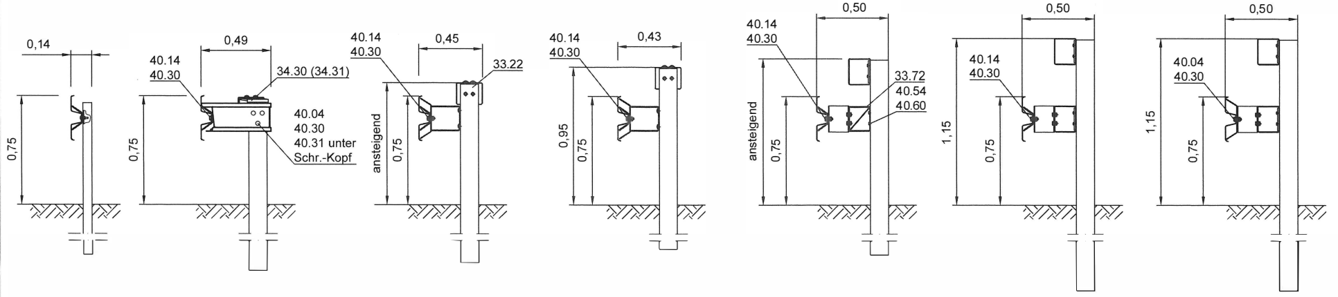
Schnitt A-A
