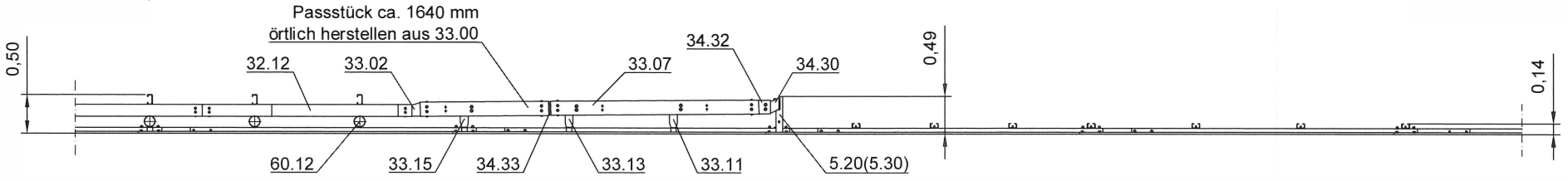
Schnitt A-A
