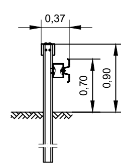
Schnitt D-D
