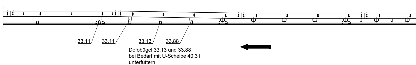
Schnitt A-A
