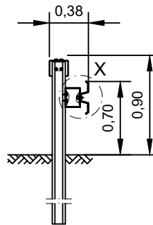
Schnitt C-C
