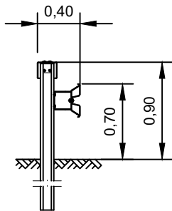
Schnitt B-B
