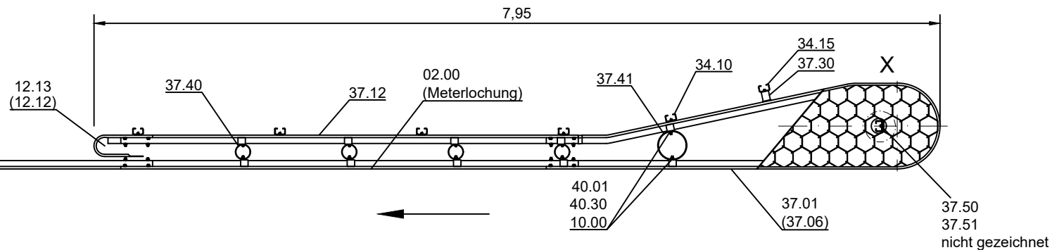
Schnitt B-B
