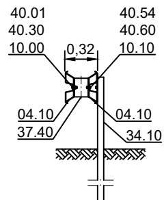
Schnitt B-B
