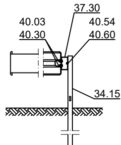
Schnitt A-A
