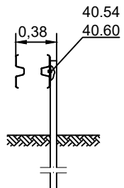
Schnitt C-C
