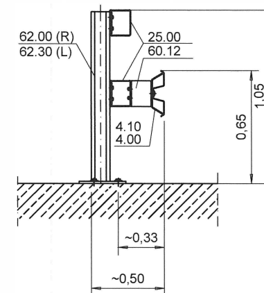
Schnitt A-A
