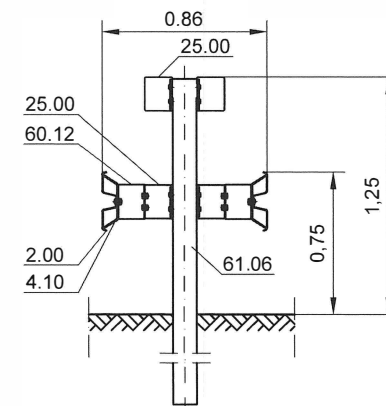
Schnitt A-A
