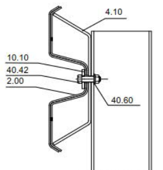
Pfostenverschraubung Profil A
