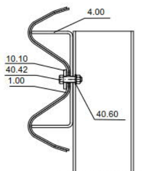
Pfostenverschraubung Profil B
