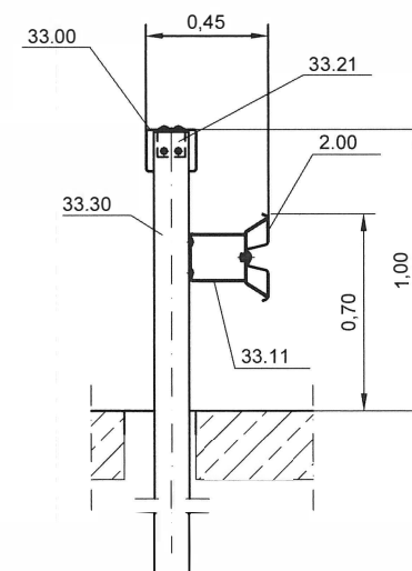
Schnitt A-A
