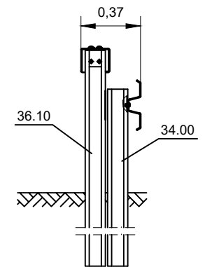
Schnitt B-B
