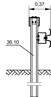
Schnitt A-A
