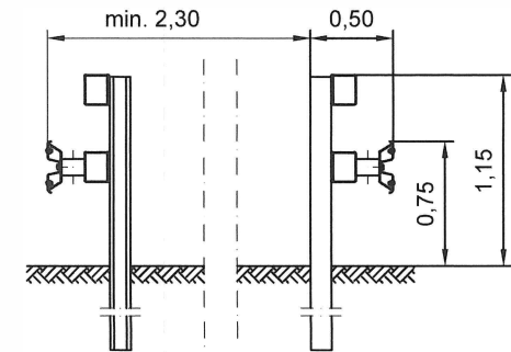
Schnitt C-C
