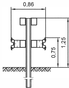
Schnitt A-A
