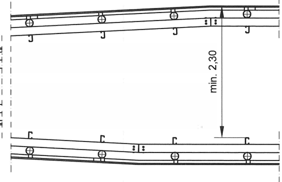
Schnitt C-C
